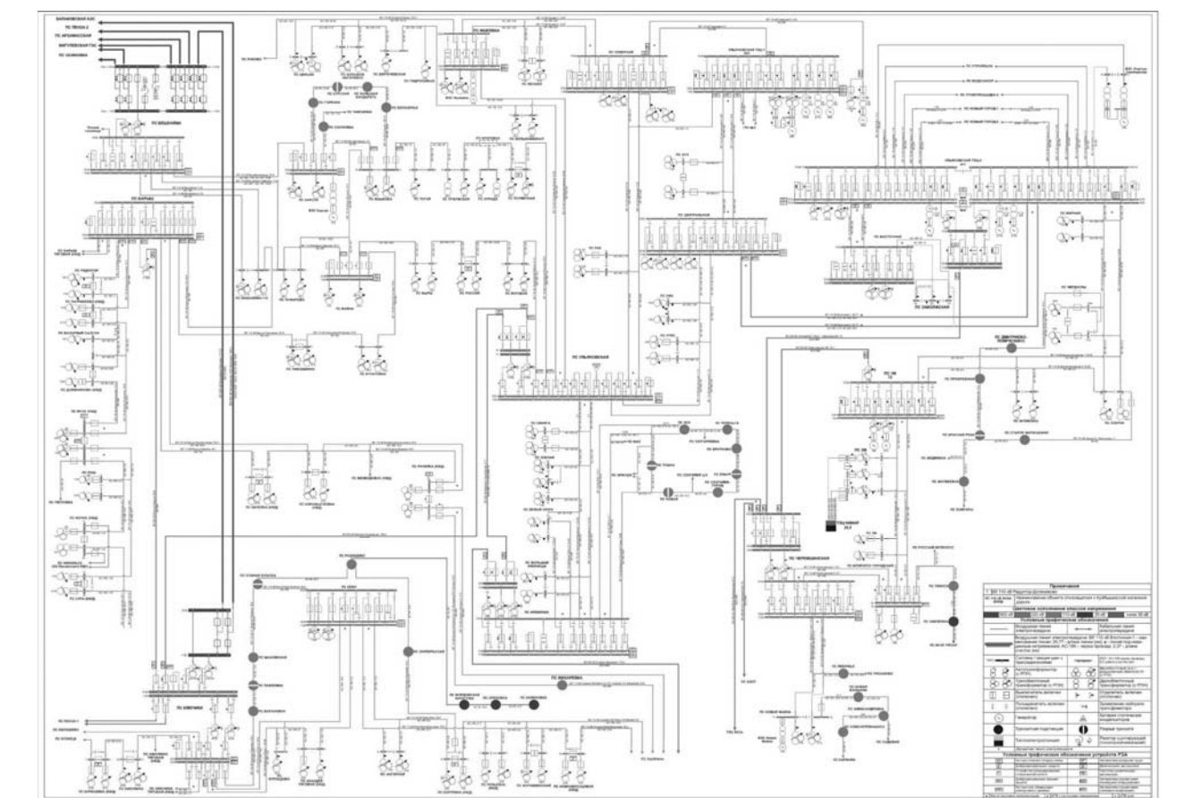
Рис. 3. Принципиальная схема электрических соединений объектов электроэнергетики энергосистемы Ульяновской области на период 2018-2022 годов
